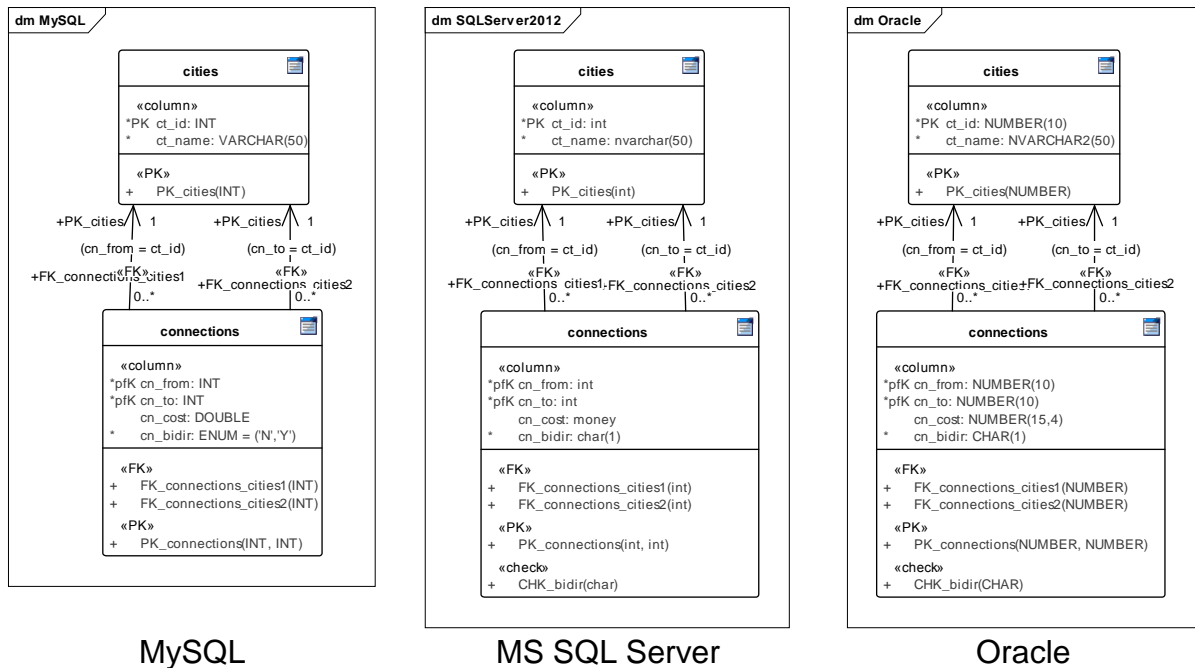
Рисунок 7.с — Таблицы cities и connections во всех трёх СУБД
