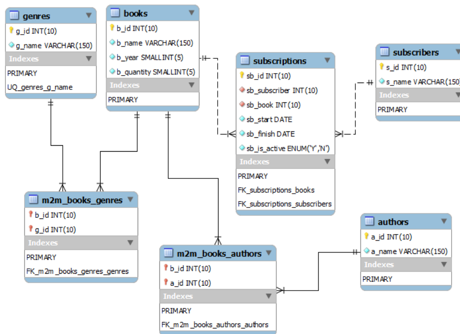
Рисунок 1.с — Модель базы данных для MySQL в MySQL Workbench
